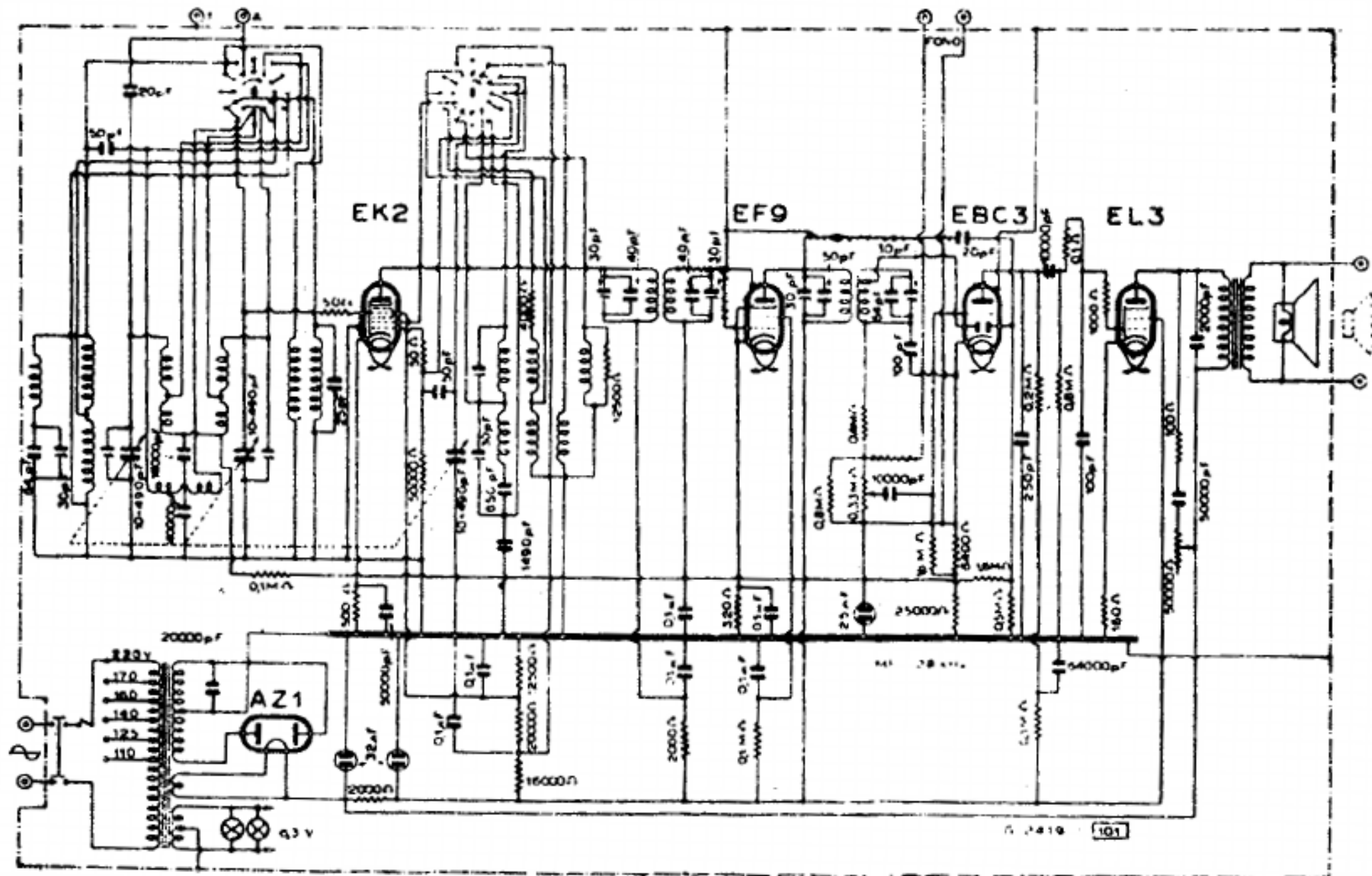
PHILIPS RADIO - MODD. « 461 E » « 469 E - FONO »
